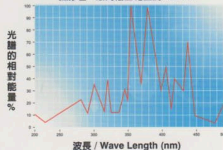
鐵摻合：最高輸出範圍到 380nm
