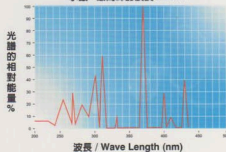
水銀：最高峰的波長 365nm
