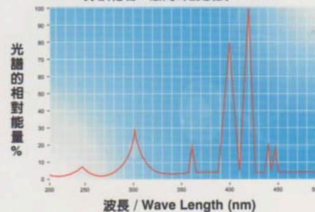
鎘鹵化物：最高峰的波長 417nm
